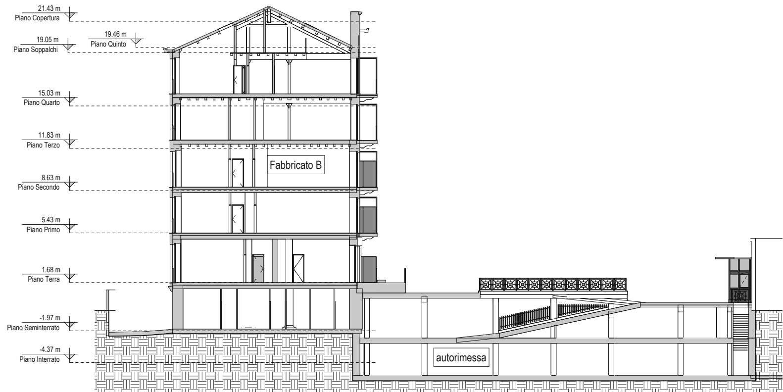
Sezione Fabbricato B
