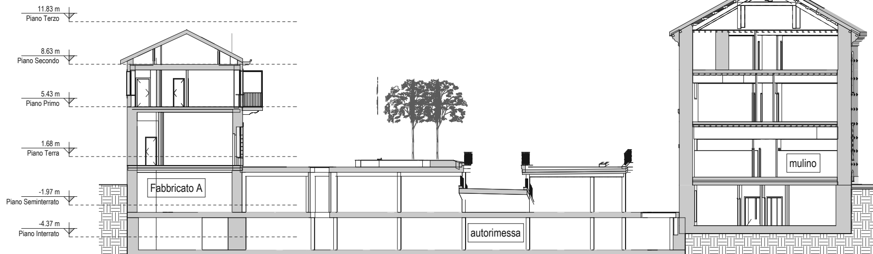
Sezione Fabbricato A
